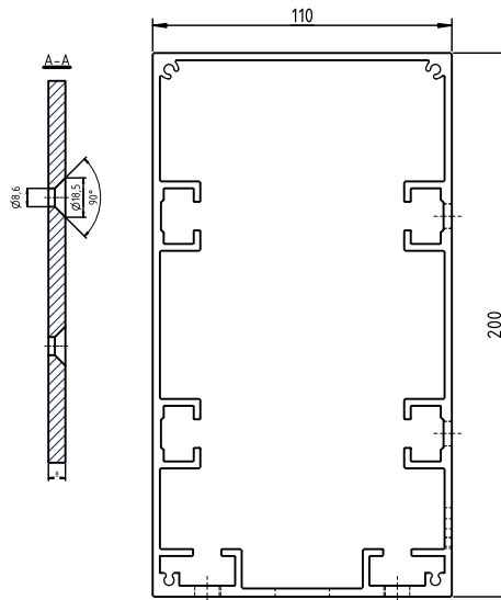
STRUKTURELL PROFIL
